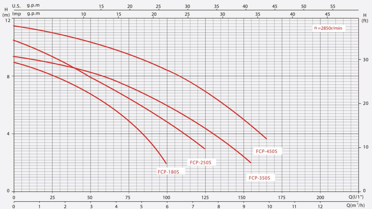
GRÁFICO DE DESEMPEÑO A n=2850 r/min
